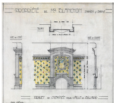
Projet d'agrandissement de la maison de l'industriel en 1924 : plan, coupe, élévation de la cheminée de la salle de billard. (Institut français d'architecture, Fonds Grenouillot Jules-André, GREAN-E-24-3) Phot. Jean-Bernard Vialles, Autr. Jules-André (architecte) Grenouillot IVR11_20089500105NUC4A
