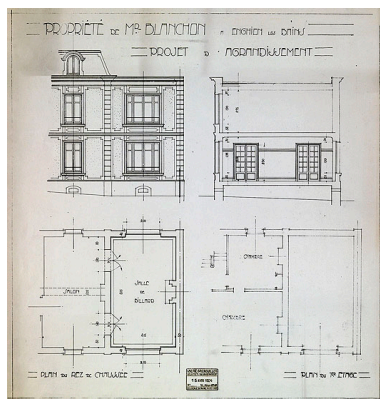
Projet d'agrandissement de la maison de l'industriel en 1924 : plans et élévation. (Institut français d'architecture, Fonds Grenouillot Jules-André, GREAN-E-24-3) Phot. Jean-Bernard Vialles, Autr. Jules-André (architecte) Grenouillot IVR11_20089500104NUC4A
