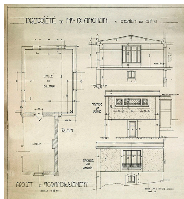
Projet d'agrandissement de la maison de l'industriel en 1924 : plan, élévations de la salle de billard et du salon. (Institut français d'architecture, Fonds Grenouillot Jules-André, GREAN-E-24-3) Phot. Jean-Bernard Vialles, Autr. Jules-André (architecte) Grenouillot IVR11_20089500106NUC4A
