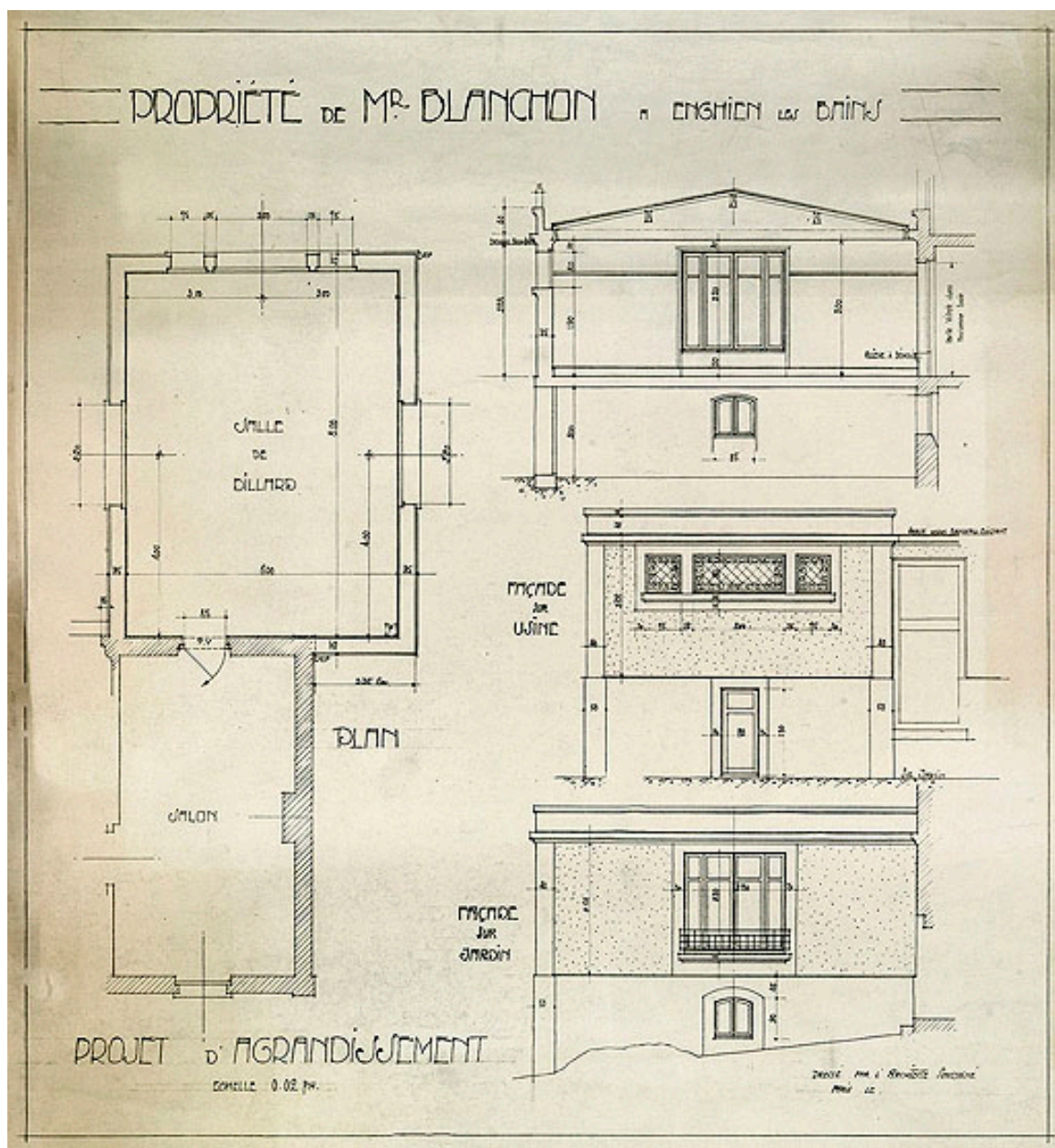
Projet d'agrandissement de la maison de l'industriel en 1924 : plan, élévations de la salle de billard et du salon. (Institut français d'architecture, Fonds Grenouillot Jules-André, GREAN-E-24-3)
