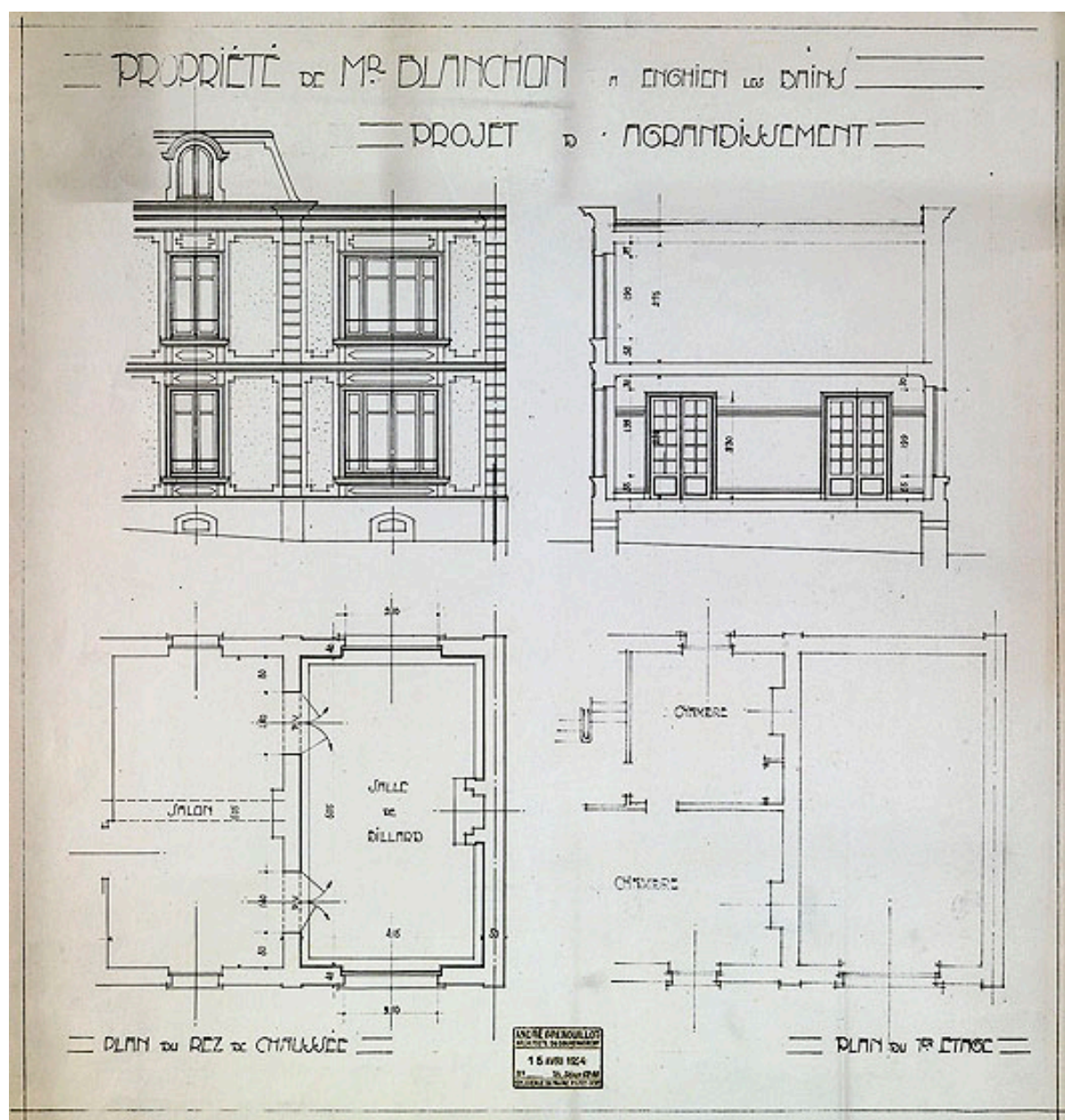
Projet d'agrandissement de la maison de l'industriel en 1924 : plans et élévation. (Institut français d'architecture, Fonds Grenouillot Jules-André, GREAN-E-24-3)
