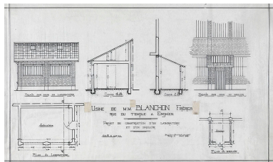
Projet d'agrandissement de l'usine en 1924 : plans, coupes, élévations d'un laboratoire et d'un brûloir. (Institut français d'architecture, Fonds Grenouillot Jules-André, GREAN-E-24-3) Phot. Jean-Bernard Vialles, Autr. Jules-André (architecte) Grenouillot IVR11_20089500107NUC4A
