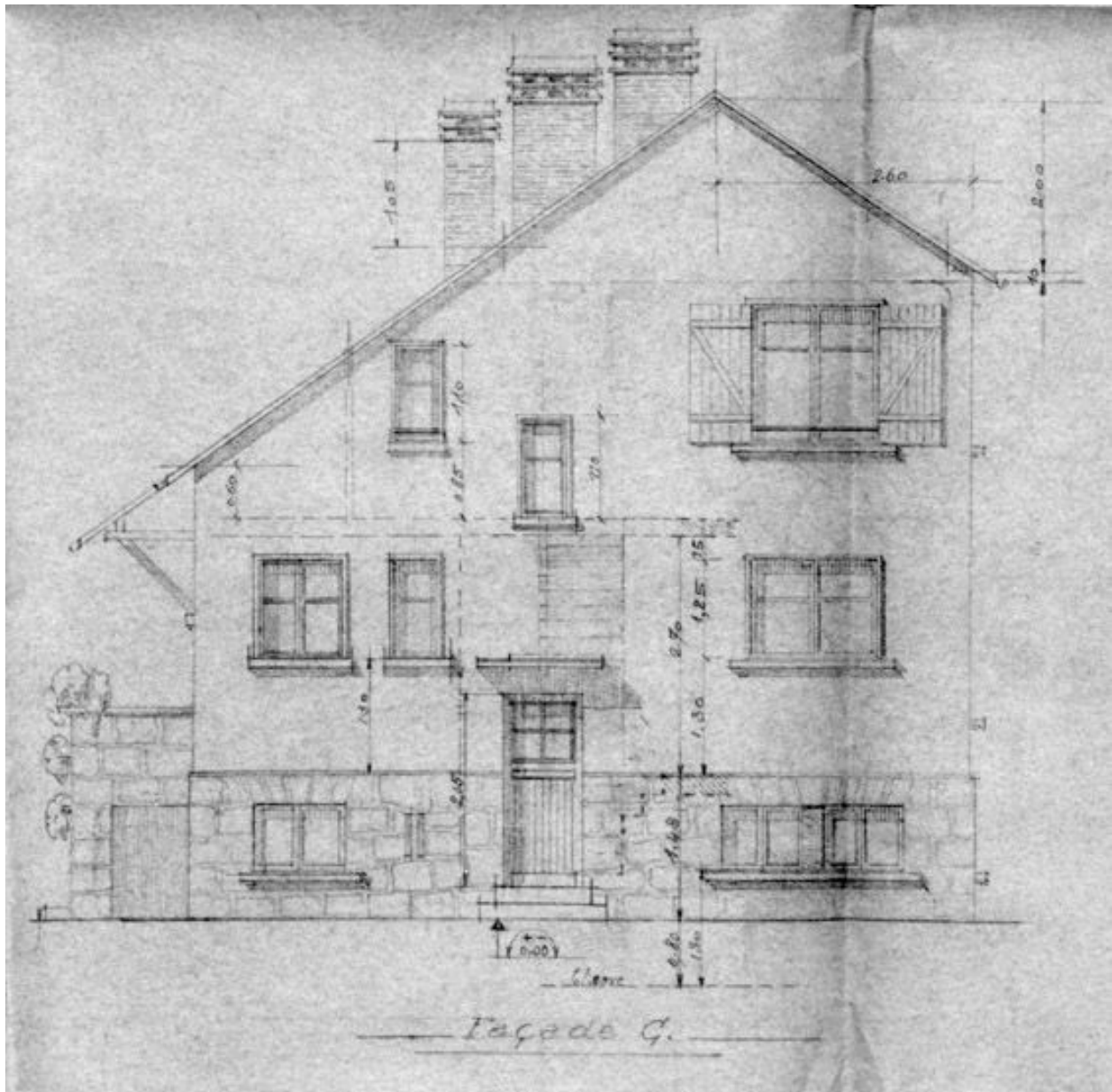
Projet de l'architecte melunais Louis Carrier pour une maison des "Castors de Melun nord" : la façade C. Tirage d'architecte, 1953. (AM Melun. 936 W 7)
