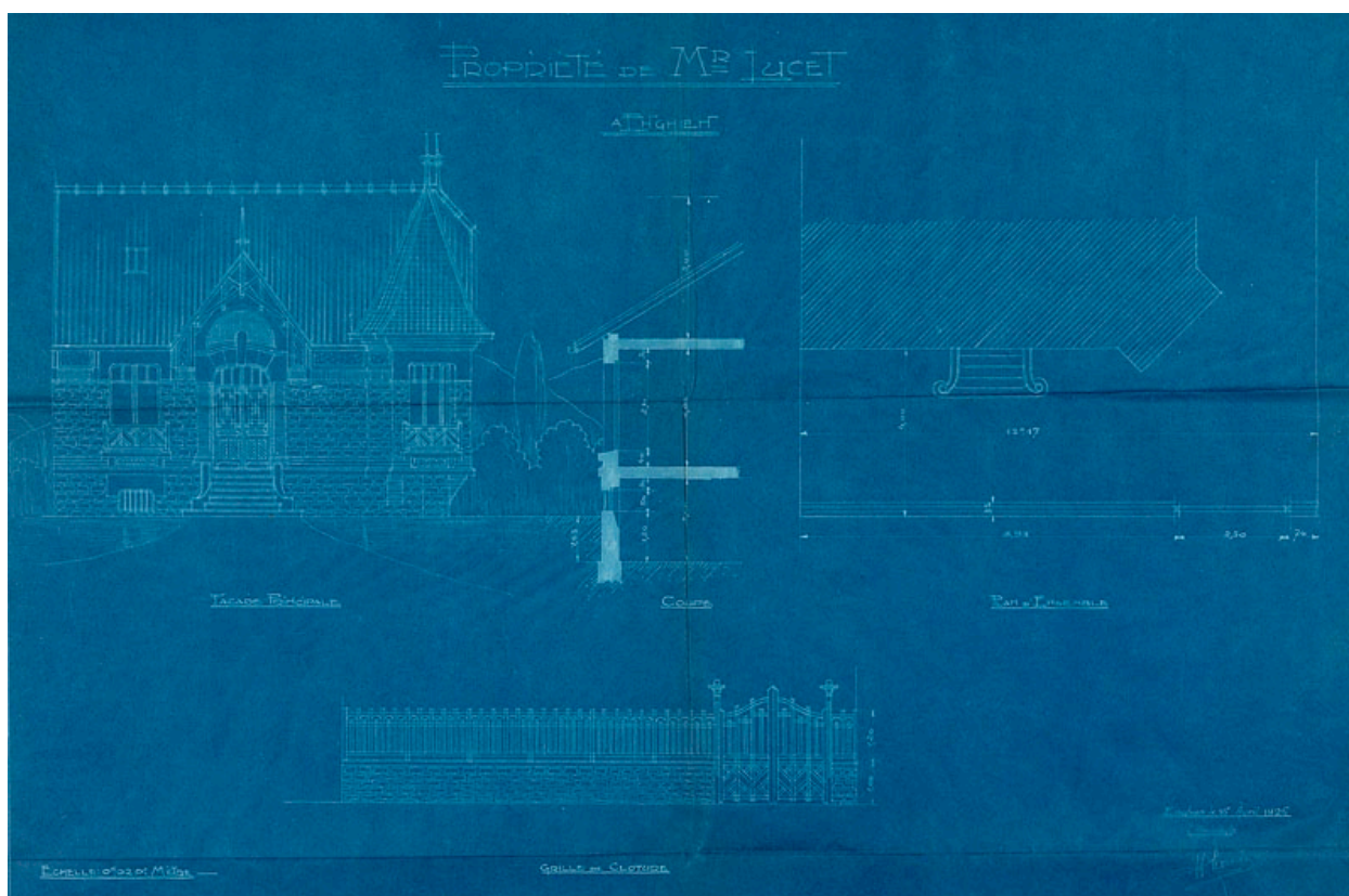
Elévation de la façade antérieure, coupe et détails de plan et de l'élévation du mur de clôture, 1926. (AM Enghien-les-Bains, 1T 134)
