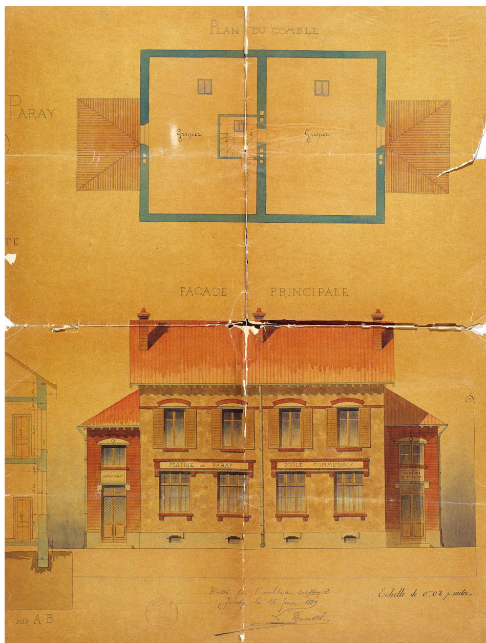
Elévation antérieure et plan du comble dessinés par l'architecte Ducastel ; Juvisy, 26 février 1889.
