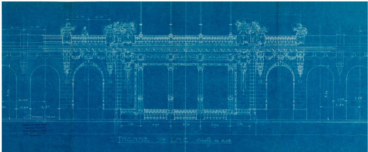
Elévation de la façade du casino donnant vers le lac. (AM Enghien-les-Bains, M109, plan n°22)
