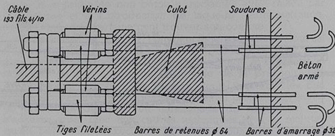
FIG. 5. — Dispositif de mise en tension d'un câble avec vérins et pompe.
