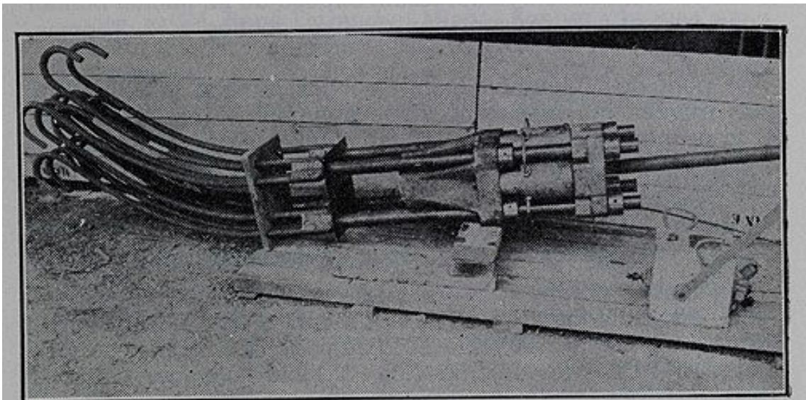
FIG. 6. — Armatures d'ancrage d'un câble.
