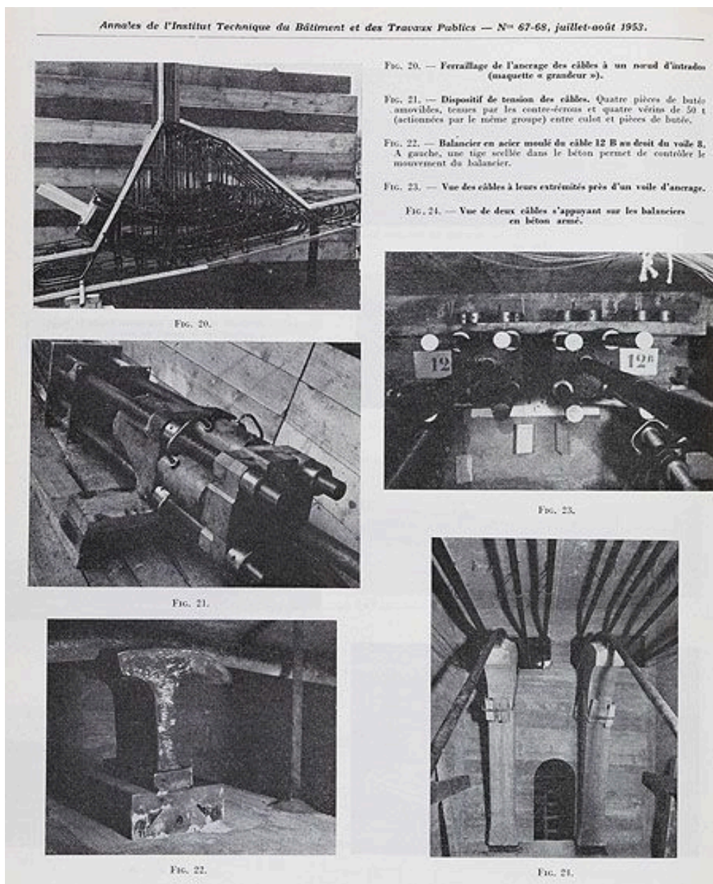
Villeneuve-Saint-Georges . Pont de Villeneuve-Saint-Georges (n°3). Différentes vues des câbles de l'ouvrage et de leur mise en oeuvre. Tiré de : Annales de l'Institut technique du bâtiment et des travaux publics, 6e année, n°67-68, juillet-août 1953.
