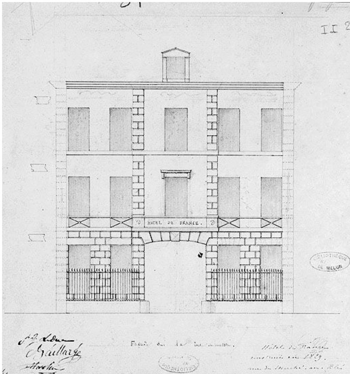
Construction de l'Hôtel de France. Façade sur la rue du Marché. Encre et crayon sur papier, 7 janvier 1829. (BM Melun. II 2)
