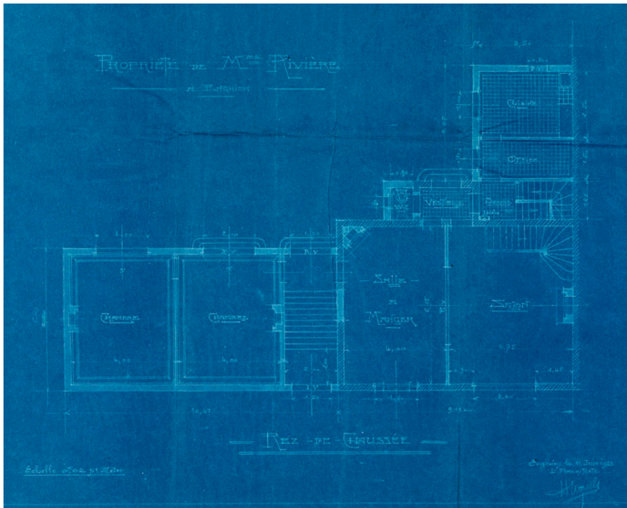
Plan du rez-de-chaussée, 1923. (AM Enghien-les-Bains, 1T 156)
