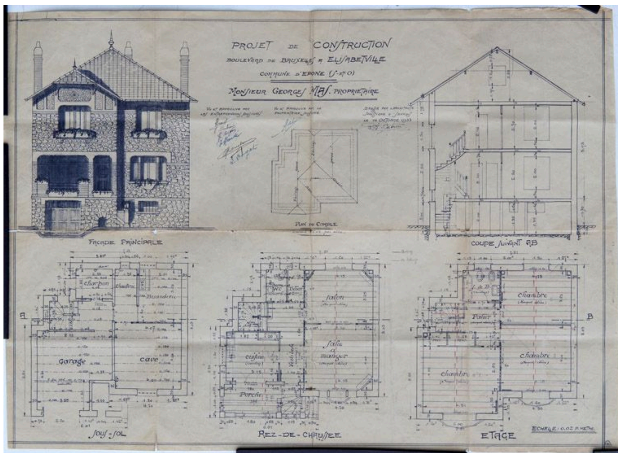
Façade, plans et coupes. Tirage. (Collection particulière).
