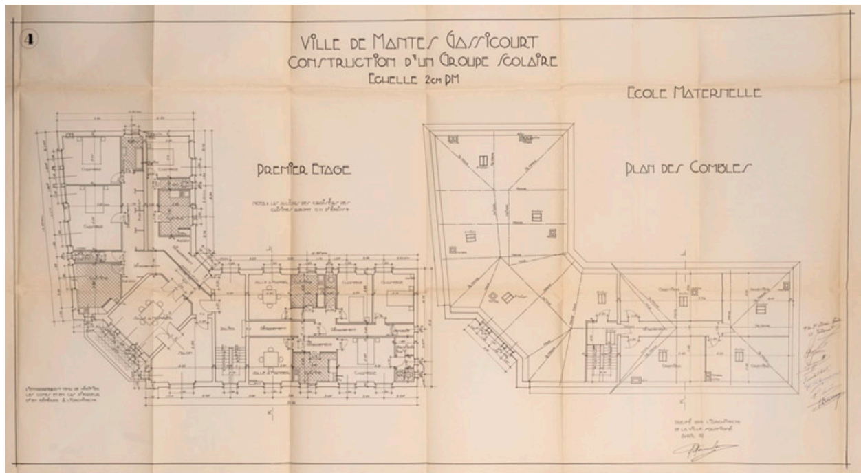
Plans du premier étage et des combles de l'école maternelle. Marabout. 1932 (AM Mantes-la-Jolie 5 M 15 (2))
