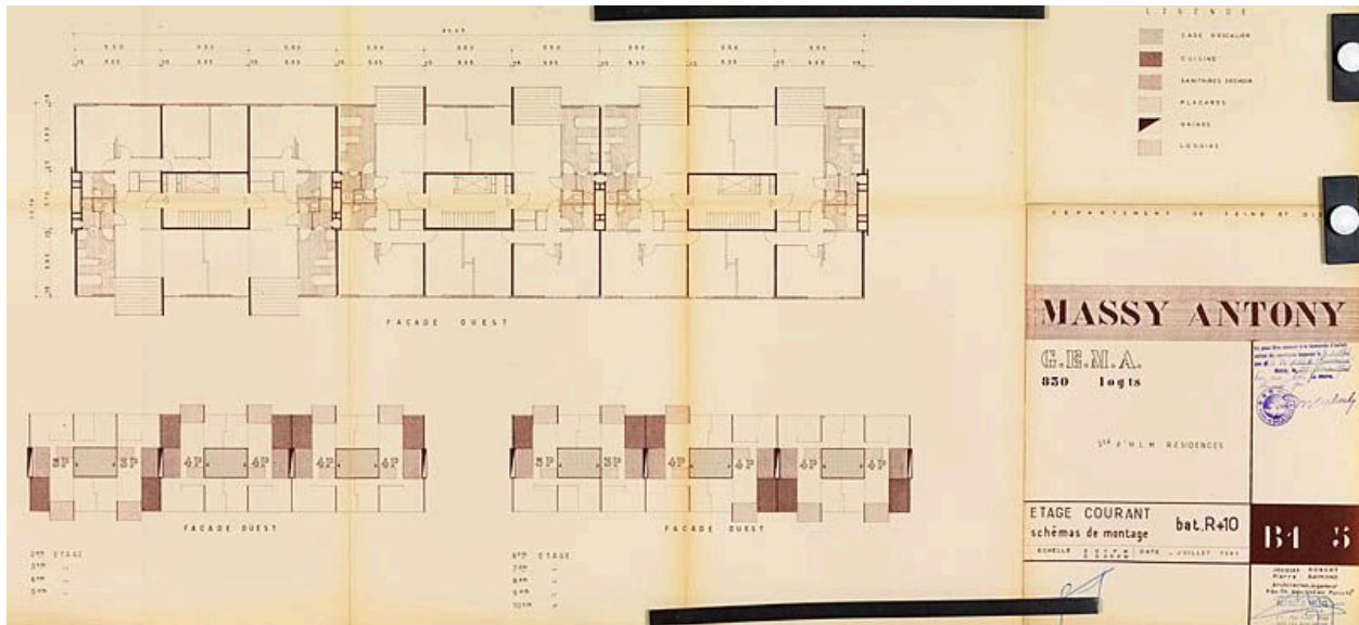
Plan d'étage courant et schéma de montage des barres R+10, juillet 1961. (AM Massy, 7 T 113)
