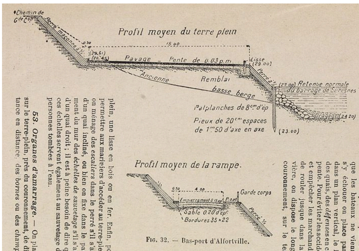
Bas port. Profil moyen du terre-plein et de la rampe. Tiré de : Notions de navigation intérieure / M. Fourrey. Paris : Ecole spéciale des travaux publics, 1929.
