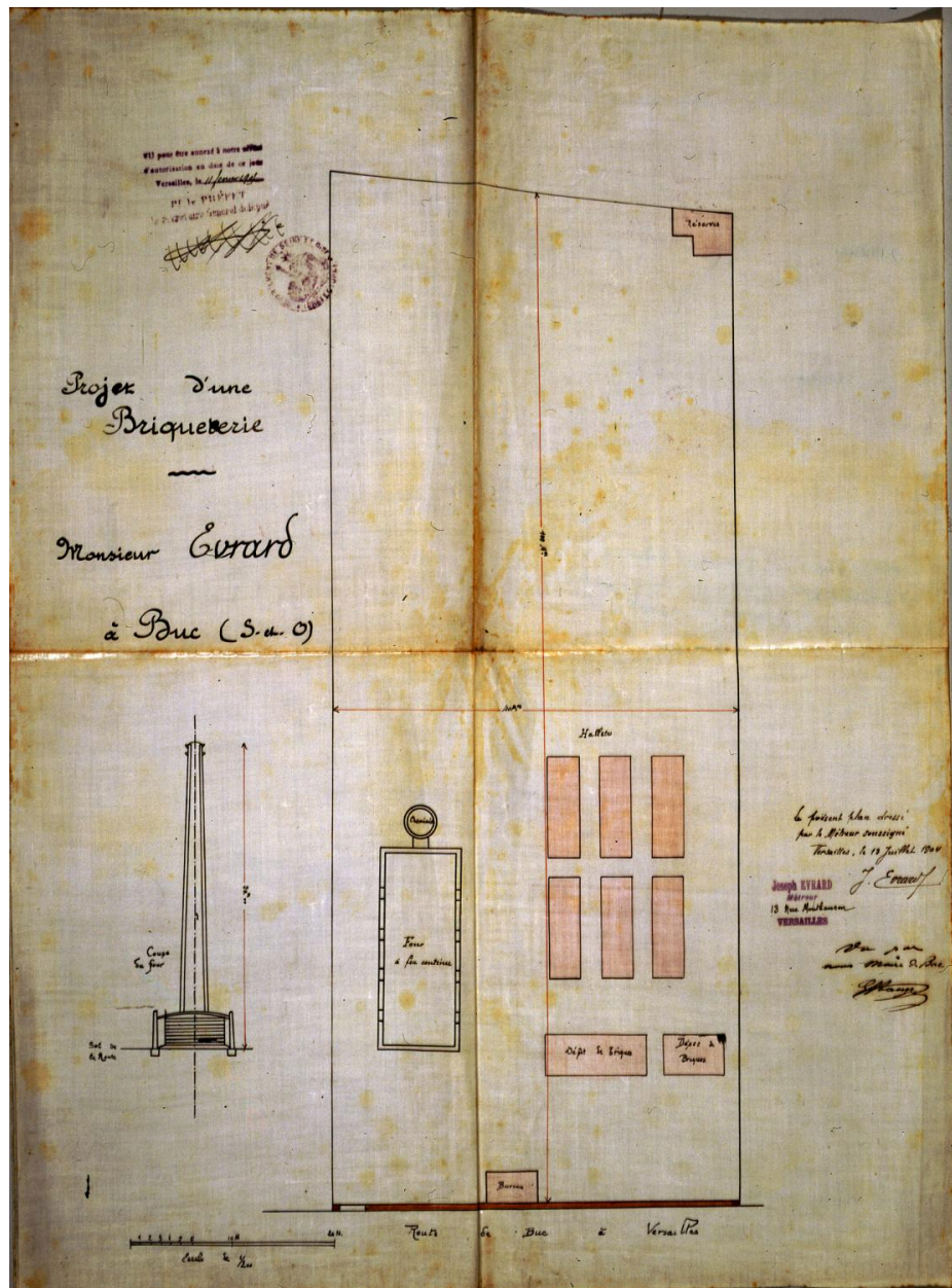
Plan de la briqueterie.
