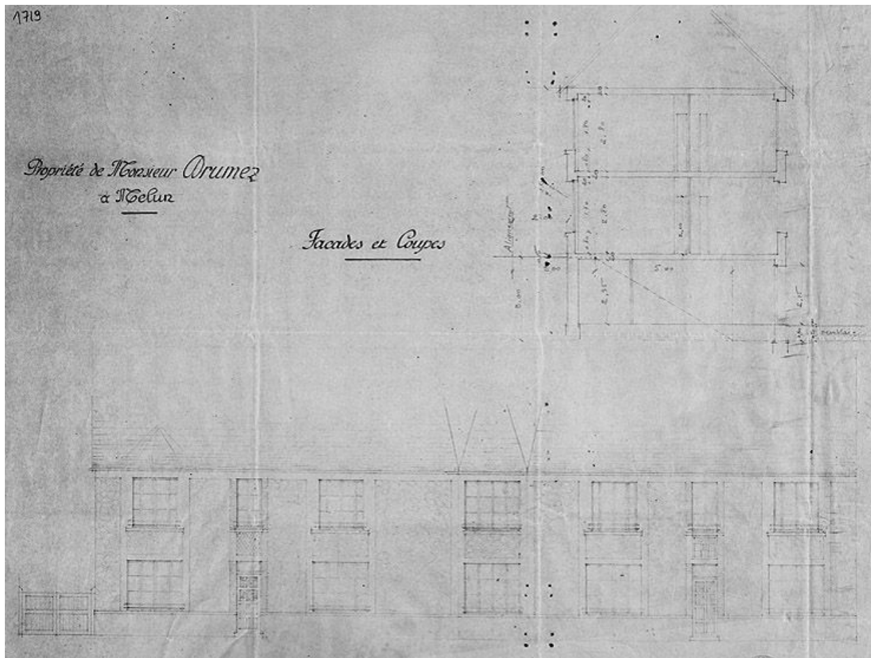
Propriété de M. Drumez à Melun, rue Poileux et rue Albert-Moreau. Façades et coupes. Papier, tirage d'architecte, 1940. (AM Melun. 1 Fi 1719)
