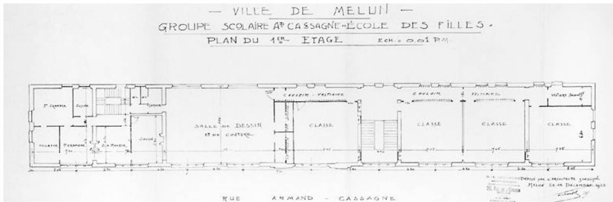
Ecole des filles : plan du premier étage. Ech 1 : 100. Papier (tirage d'architecte), 12 décembre 1922. (AM Melun. 1 Fi 723)
