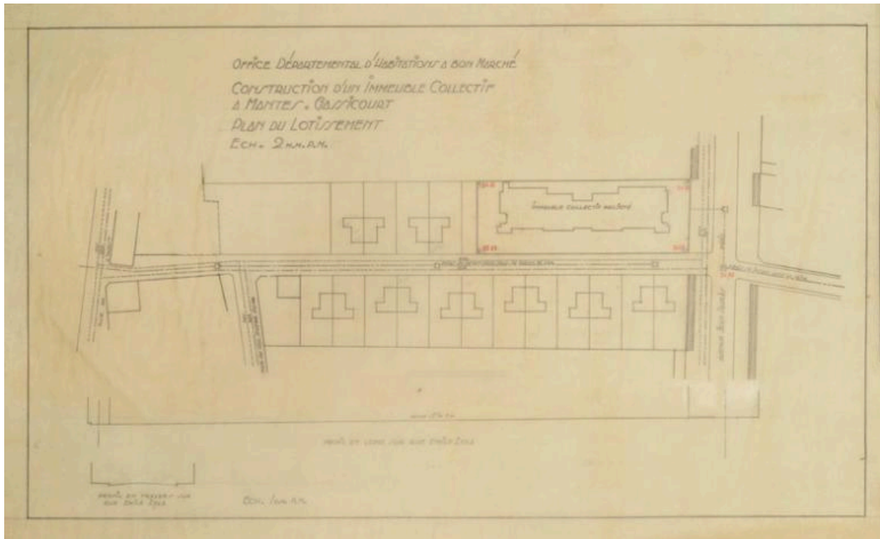
Plan masse du lotissement comprenant habitat collectif et individuel. AM Mantes-la-Jolie (non coté).
