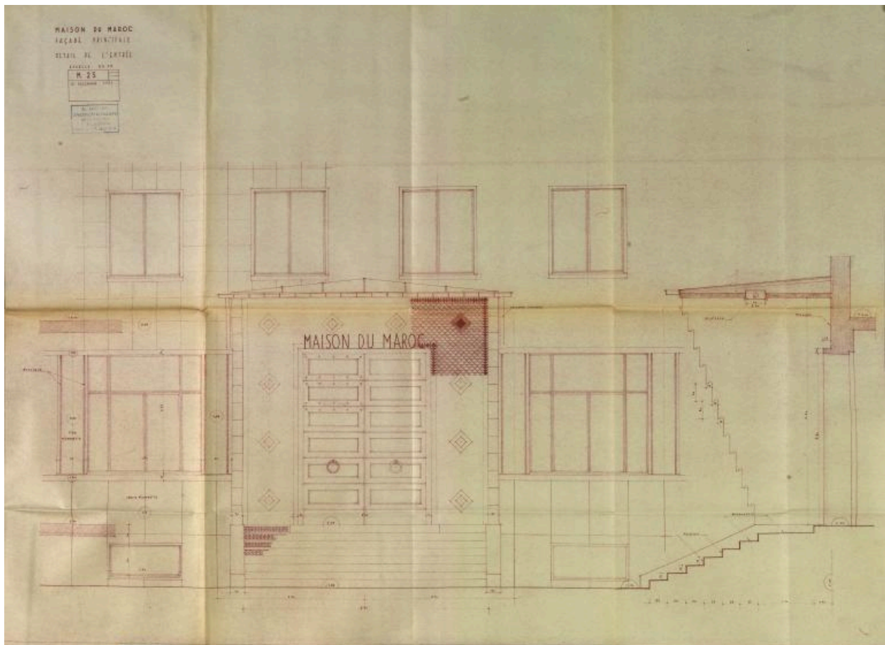
Façade principale : détail de la porte d'entrée sur le boulevard Jourdan ; A. Laprade, J. Vernon, B. Philippe, architectes ; 15 décembre 1951. Plan. Archives nationales, 20090013/393.
