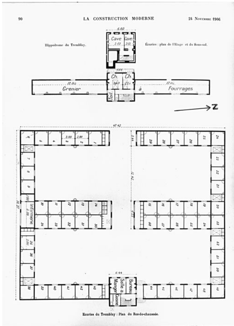
Plan du rez-de-chaussée des écuries. Tiré de : La construction moderne, 1906-1907.
