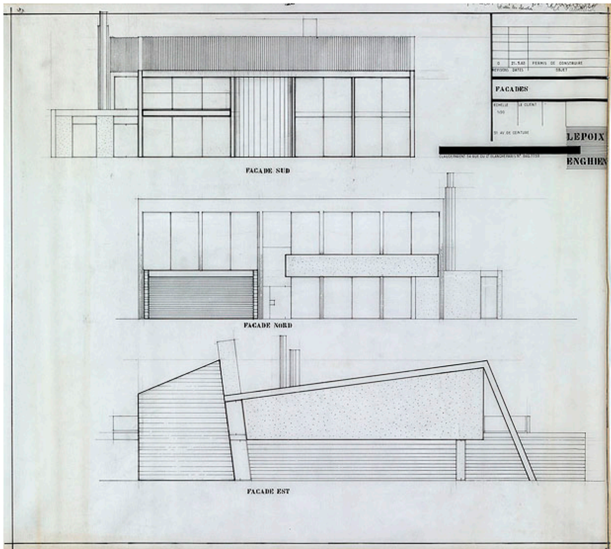
Projet de Claude Parent : élévations des façades sud, nord, est, 1963. (Institut français d'architecture, Fonds Parent Claude, PARCL-B-63-01)
