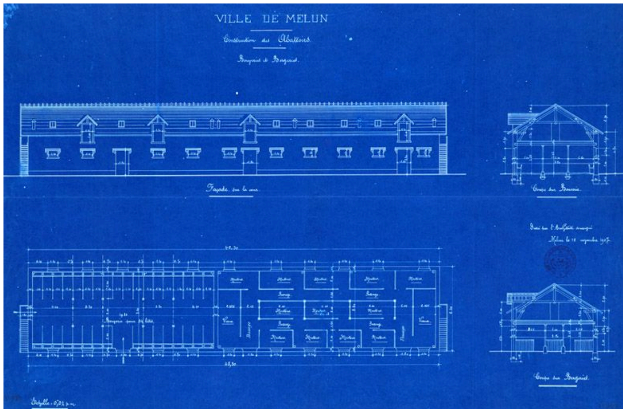
Ville de Melun. Construction des abattoirs. Bouveries et bergeries (12 novembre 1907). (complément du Doc. 8). Projet non réalisé. Papier, bleu, 1907. (AM Melun. 1 Fi 1599)
