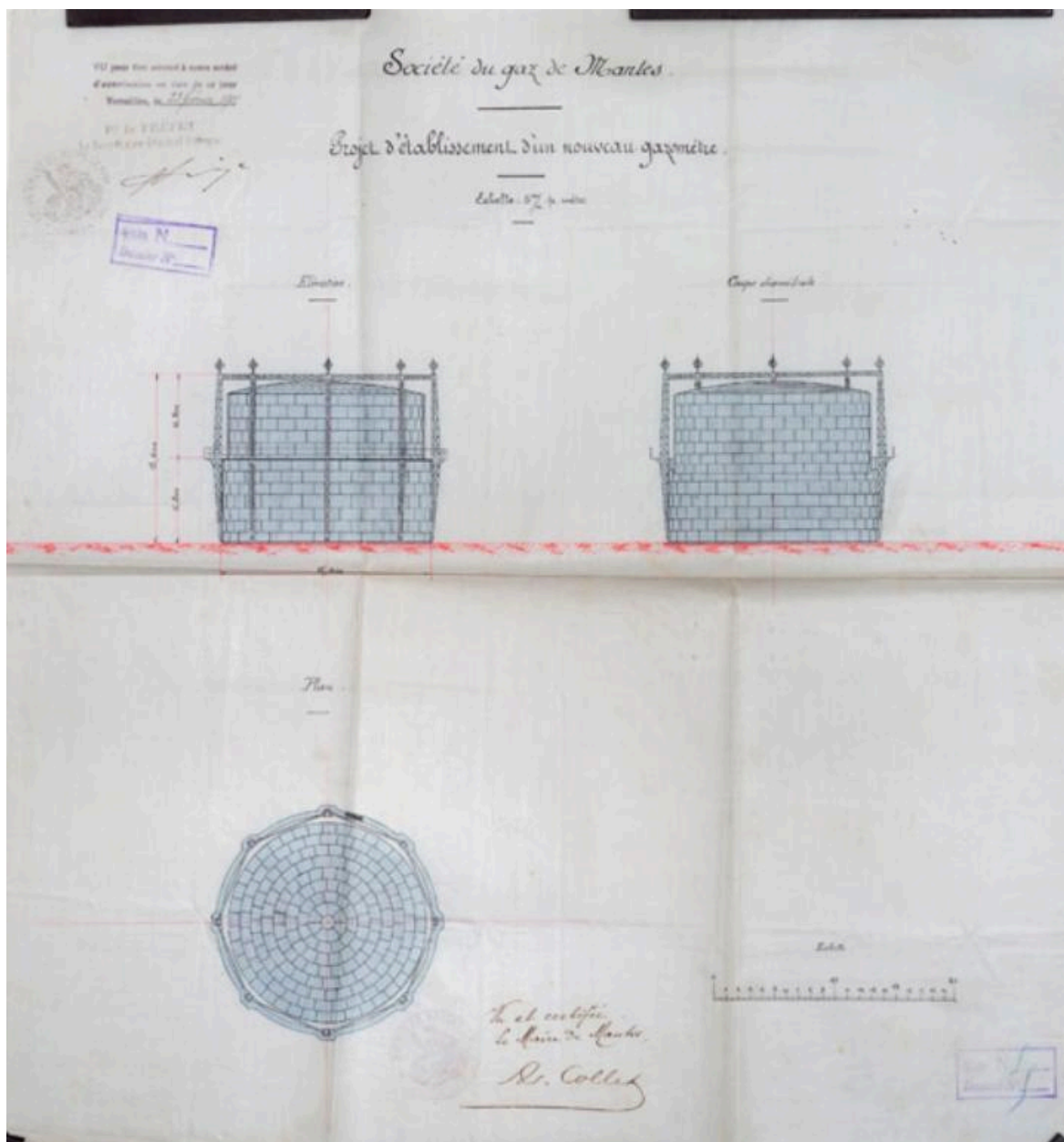
Plan, coupe et élévation du gazomètre projeté en 1901. AM Mantes-la-Jolie, 4 O 13
