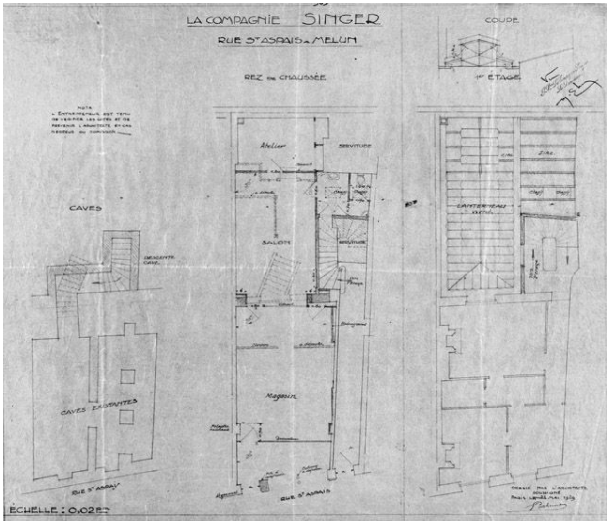
Plan du rez-de-chaussée, sous-sol et premier étage, coupe de l'immeuble, 8 rue Saint-Aspais. Tirage d'architecte, 1929 (8 mai). (AM Melun. 1 Fi 969)
