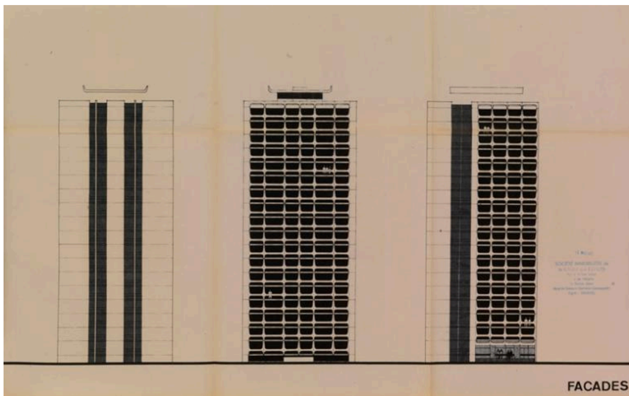
Quartier 1. Nouveau projet de tours par H. Longepierre. Façades. 1969. Mantes-la-Jolie. Permis de construire. 36/69
