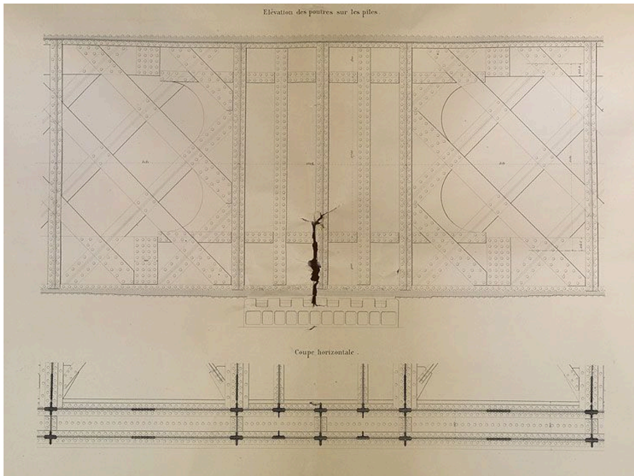
Choisy-le-Roi. Pont ferroviaire de la Grande Ceinture. Elévation des poutres sur les piles. (Ecole nationale des ponts et chaussées)
