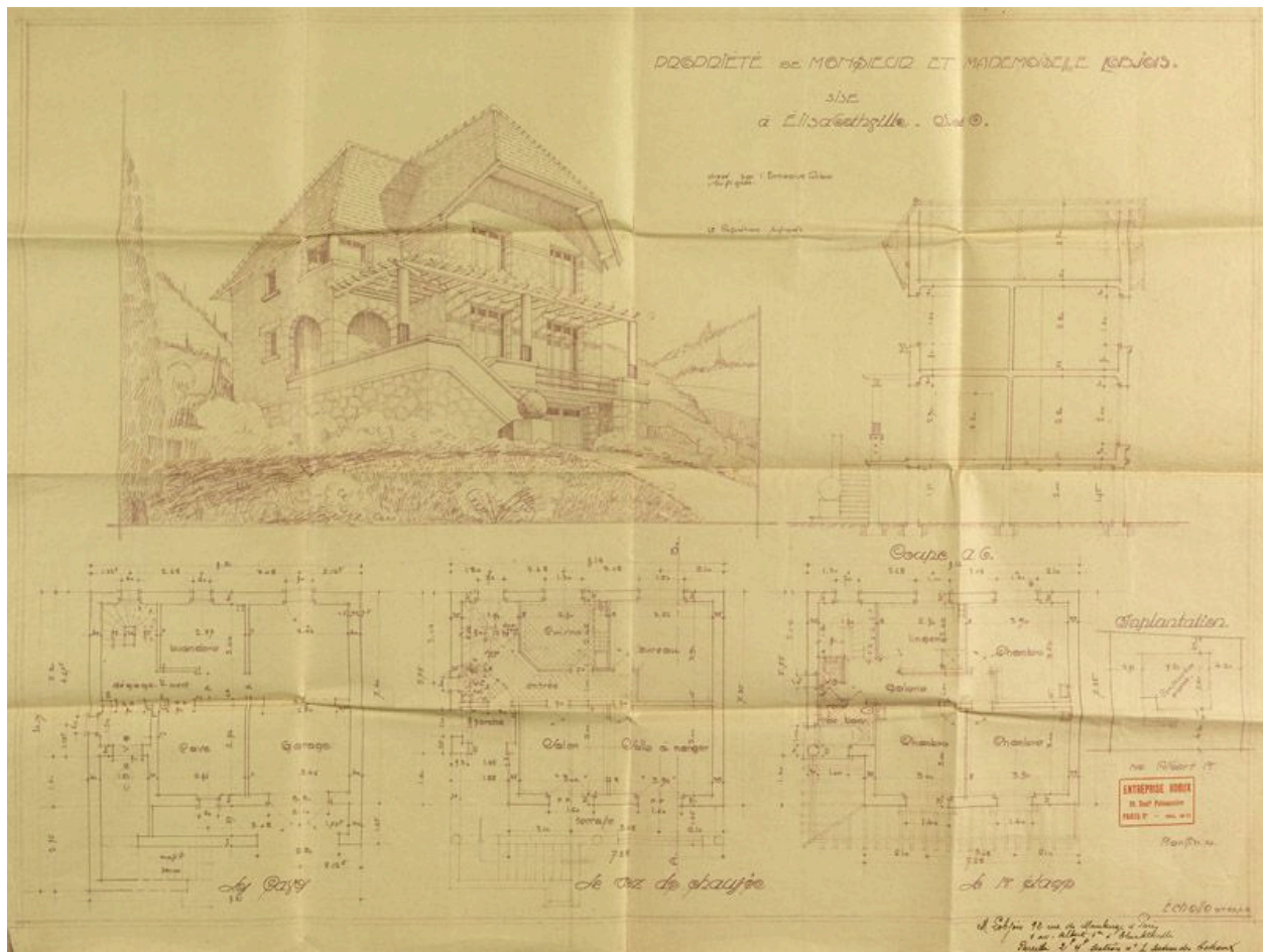
Façade et plans de la maison. Tirage (Archives municipales Aubergenville)
