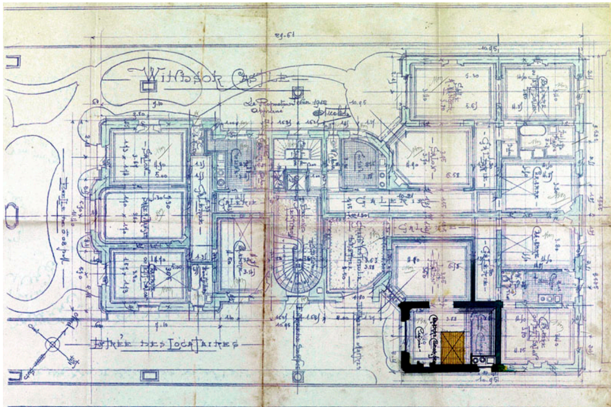
Plan du rez-de-chaussée (1912). (AM Enghien-les-Bains, 1T 65)
