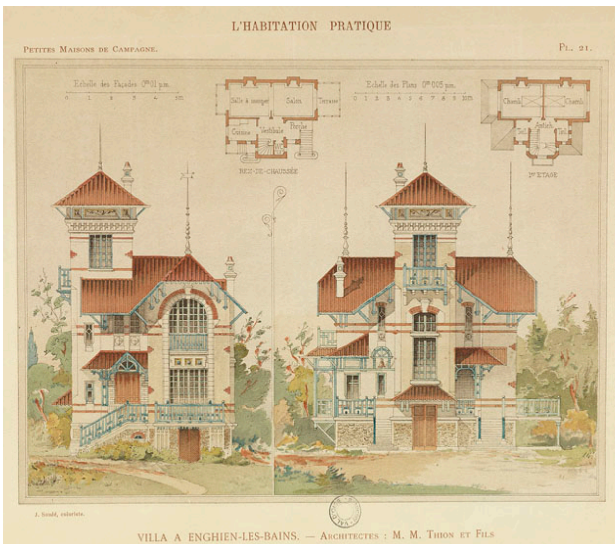
Elévations, plans du rez-de-chaussée et du premier étage, 1904. (AD Val d'Oise, 20Fi 59/19-230, en feuillet détaché)
