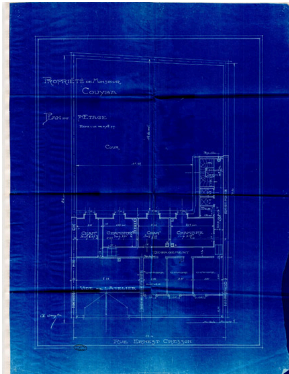
Plan du 7e étage.-Plan, 1913. (Archives de Paris VO 11 1131).
