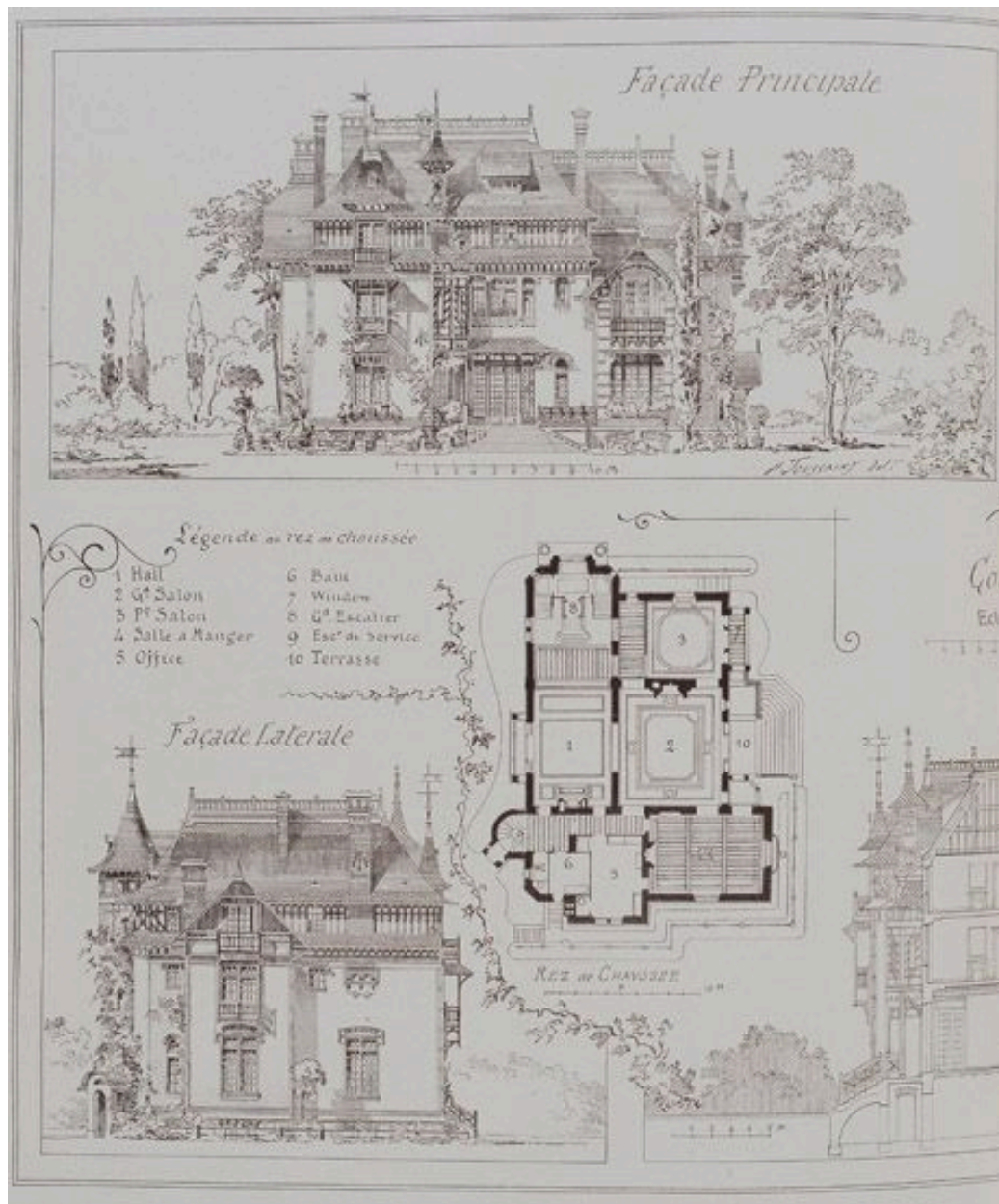
Façades principale et latérale, plan du rez-de-chaussée. Plan et élévations. Tiré de : La Construction moderne, 1891-1892. (BHVP, Per F° 303)
