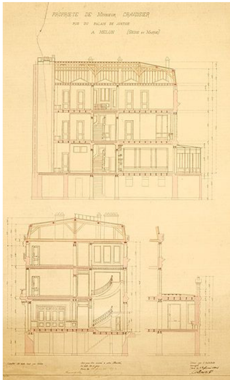
Propriété de M. Cravoisier, rue du Palais de Justice, coupes longitudinale et transversale. Papier, 1893. (AM Melun. 1 Fi 1638)
