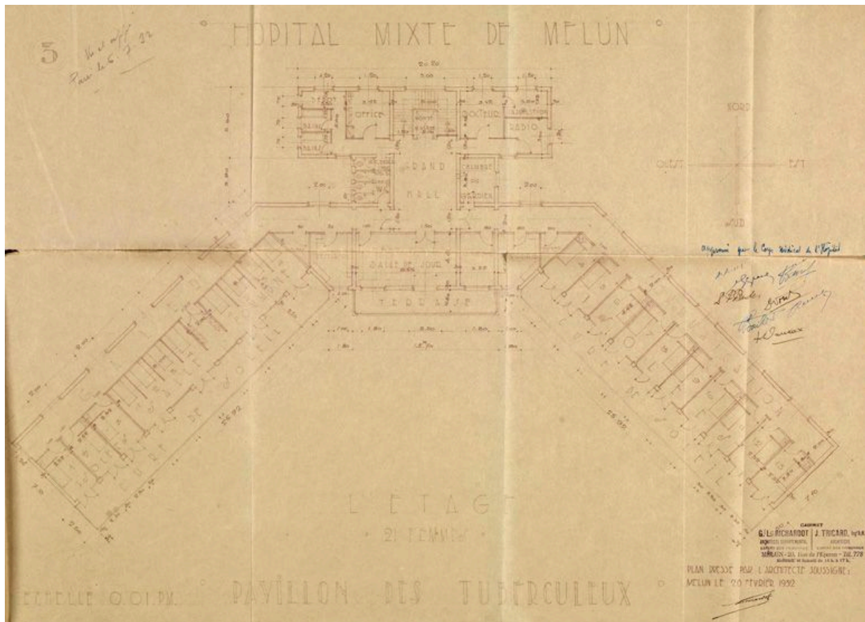
Projet de construction du sanatorium : plan de l'étage, 12 mars 1932. (AD Seine-et-Marne. Série X (cotation en cours lors de l'étude))
