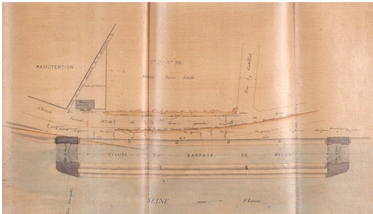
Plan de l'écluse. Calque aquarellé, 23 août 1872. (AD Seine-et-Marne. Op 3302)
