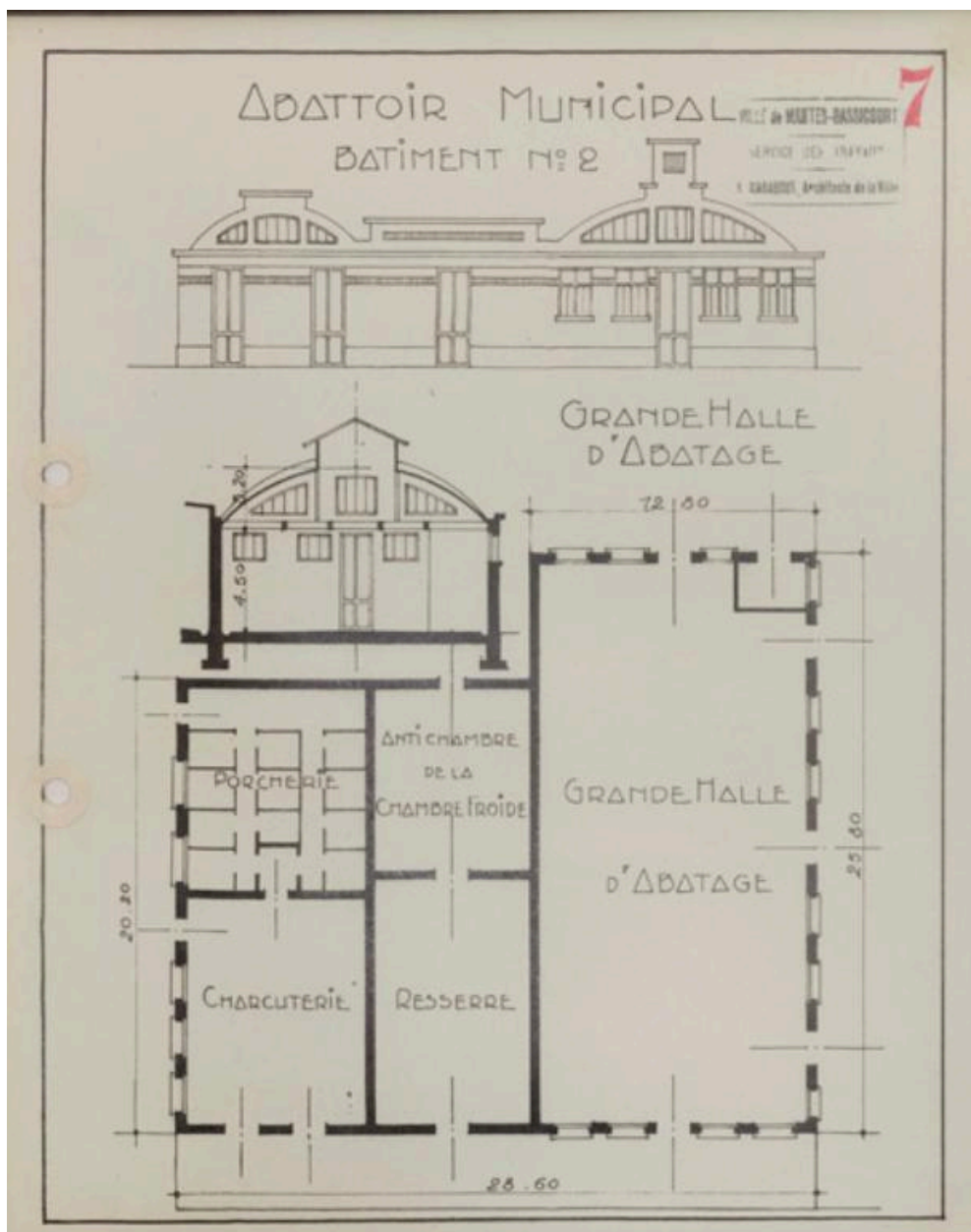
Elévation et plan de la grande halle d'abattage vers 1940. AM. Mantes-la-Jolie, 1 M 1.
