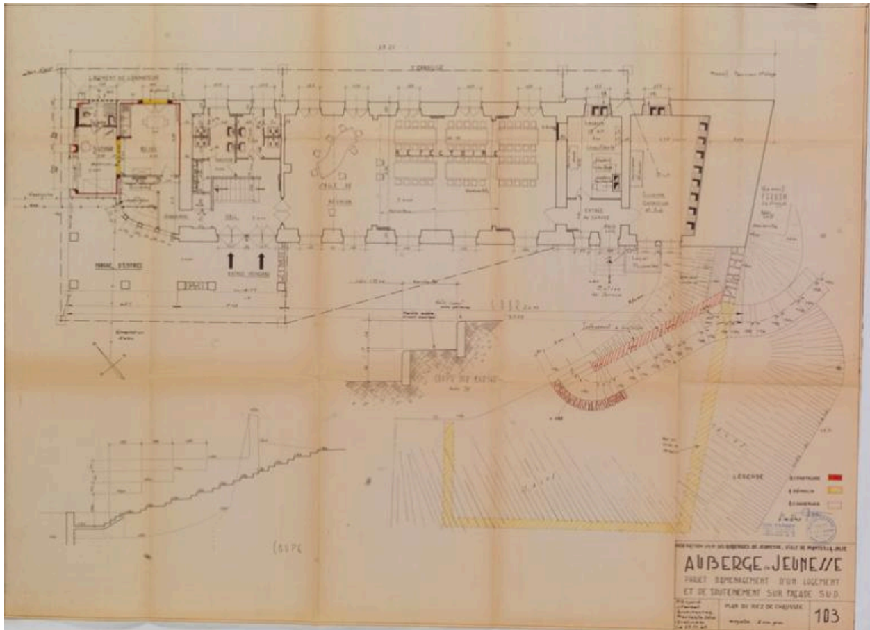
Aménagement de l'ancien couvent des Cordeliers en auberge de jeunesse, plan du rez-de-chaussée, 1965, M. Gojard, J. Perbet (AM Mantes-la-Jolie 5M).
