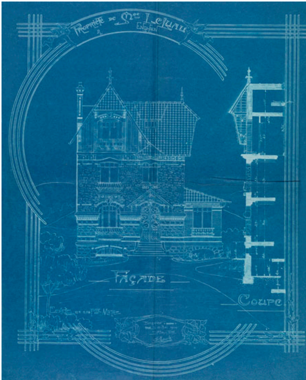
Elévation et coupe d'une maison construite pour madame Le Luau en 1914 (non localisée). (AM Enghien-les-Bains, Fonds des autorisations de permis de construire)
