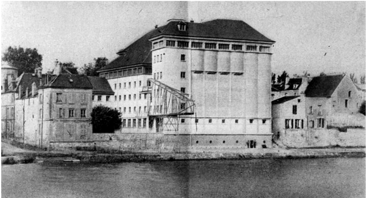
Vue d'ensemble, côté Seine. Tiré de : Les nouveaux Moulins de Melun, dans La Meunerie française, n° 27, septembre 1948. (Conservatoire national des arts et métiers. Pt Fol Ku 17)
