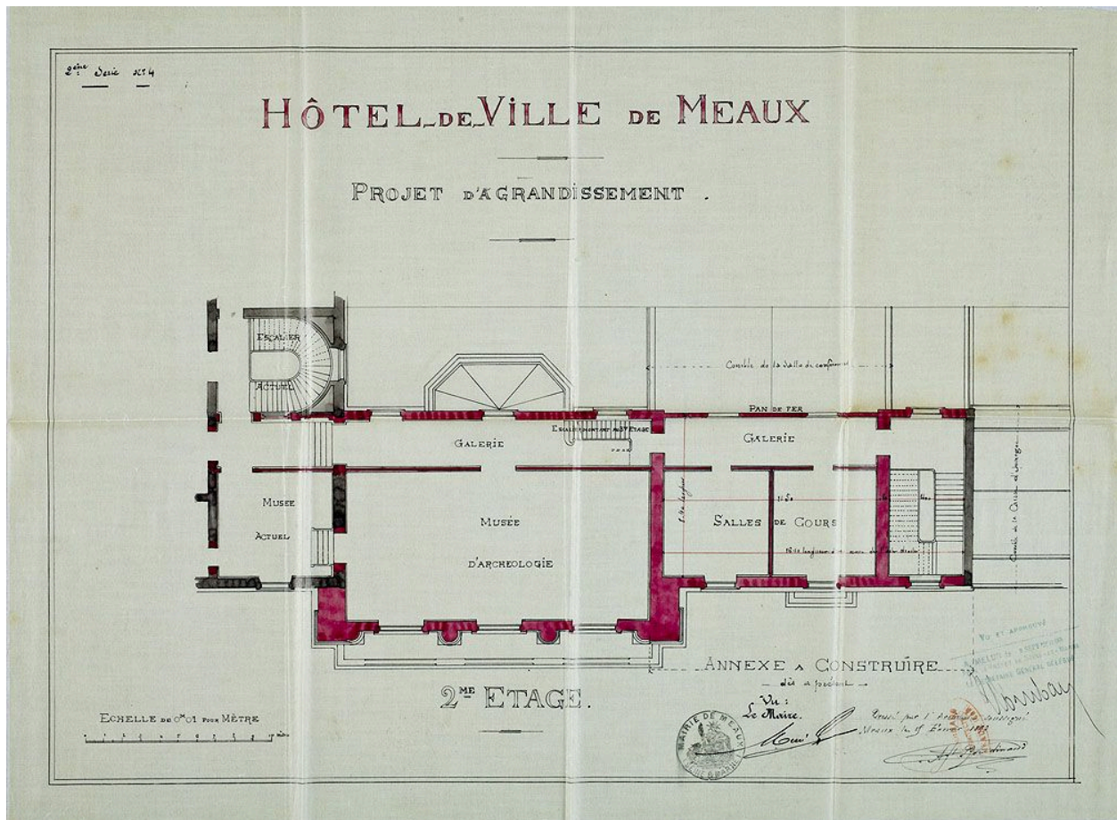
Projet d'agrandissement, 1893 : plan du 2ème étage. Encre sur calque. (AD Seine-et-Marne. 4 Op 284/17)
