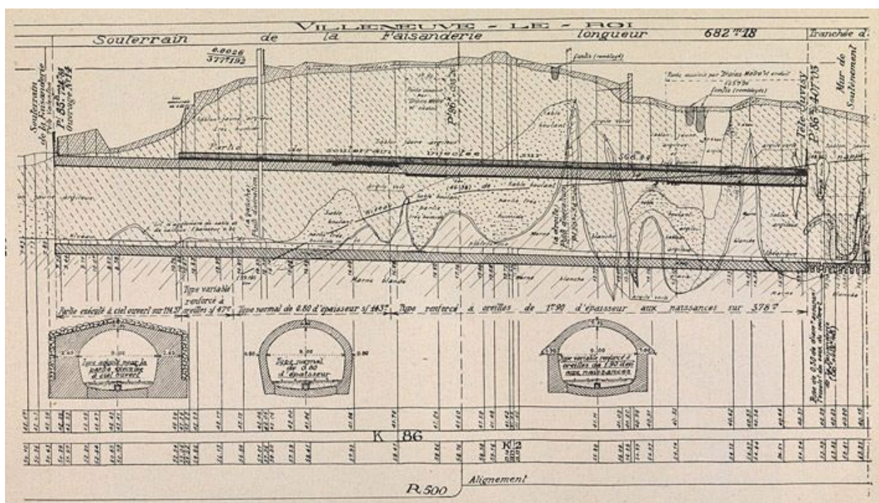
Voie ferrée dit raccordement de Valenton de la ligne de Grande Ceinture. Détail du souterrain de la faisanderie à Villeneuve-le-Roi. Tiré de : Le raccordement de Valenton/ M. Habouzit. In Revue Générale des Chemins de Fer, 1er mai 1938, p. 287-298.
