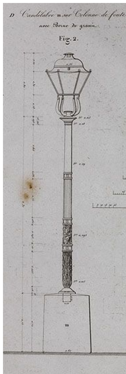
Ivry-sur-Seine. Pont d'Ivry (n°1). Détail d'un candélabre. Tiré de : Pont d'Ivry en bois, sur piles en pierre, traversant la Seine... / MHC Emmery. Paris : Carilian-Goeury, 1832. (Ecole nationale des ponts et chaussées)
