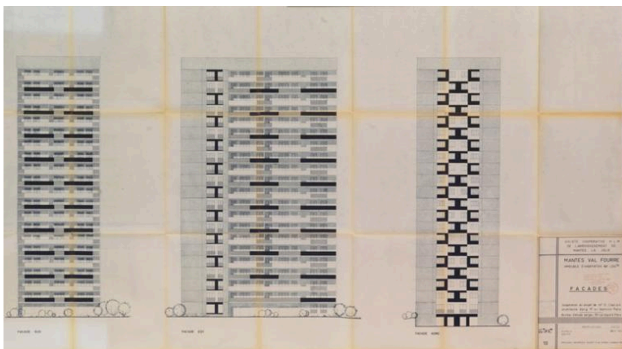
Quartier 2. La tour "Véga". Façades. 1964. Mantes-la-Jolie. Permis de construire 51/63.
