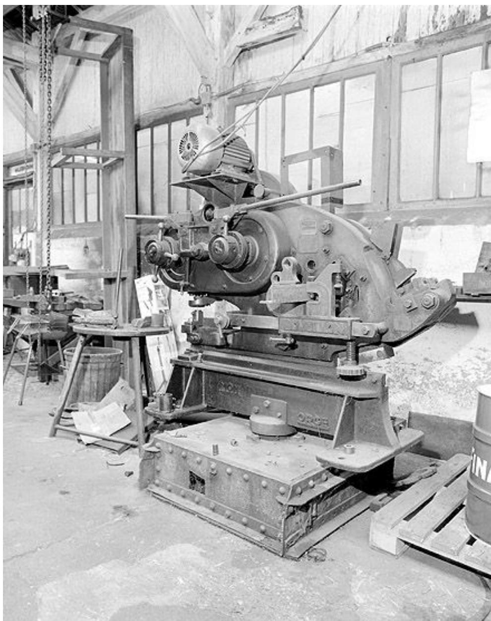
Coupe fer, poinçonneuse : vue générale de la machine.
