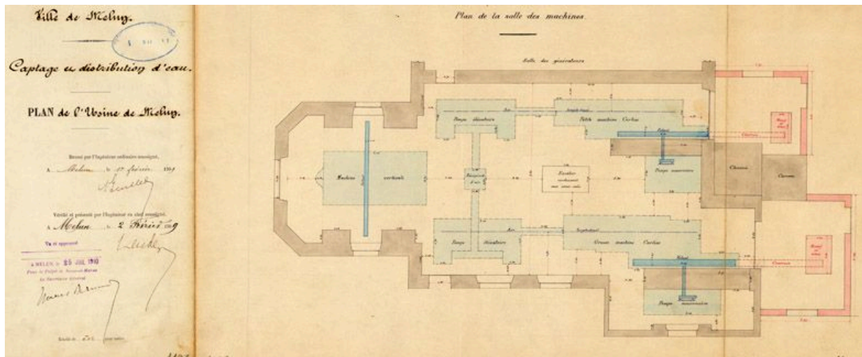
Plan de l'usine de captage et distribution d'eau de Melun : la salle des machines, 1er février 1909. (AM Melun. 1 Fi 1197)
