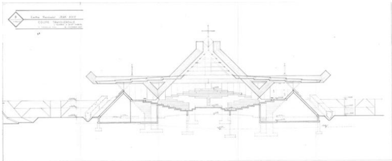
Coupe transversale.
