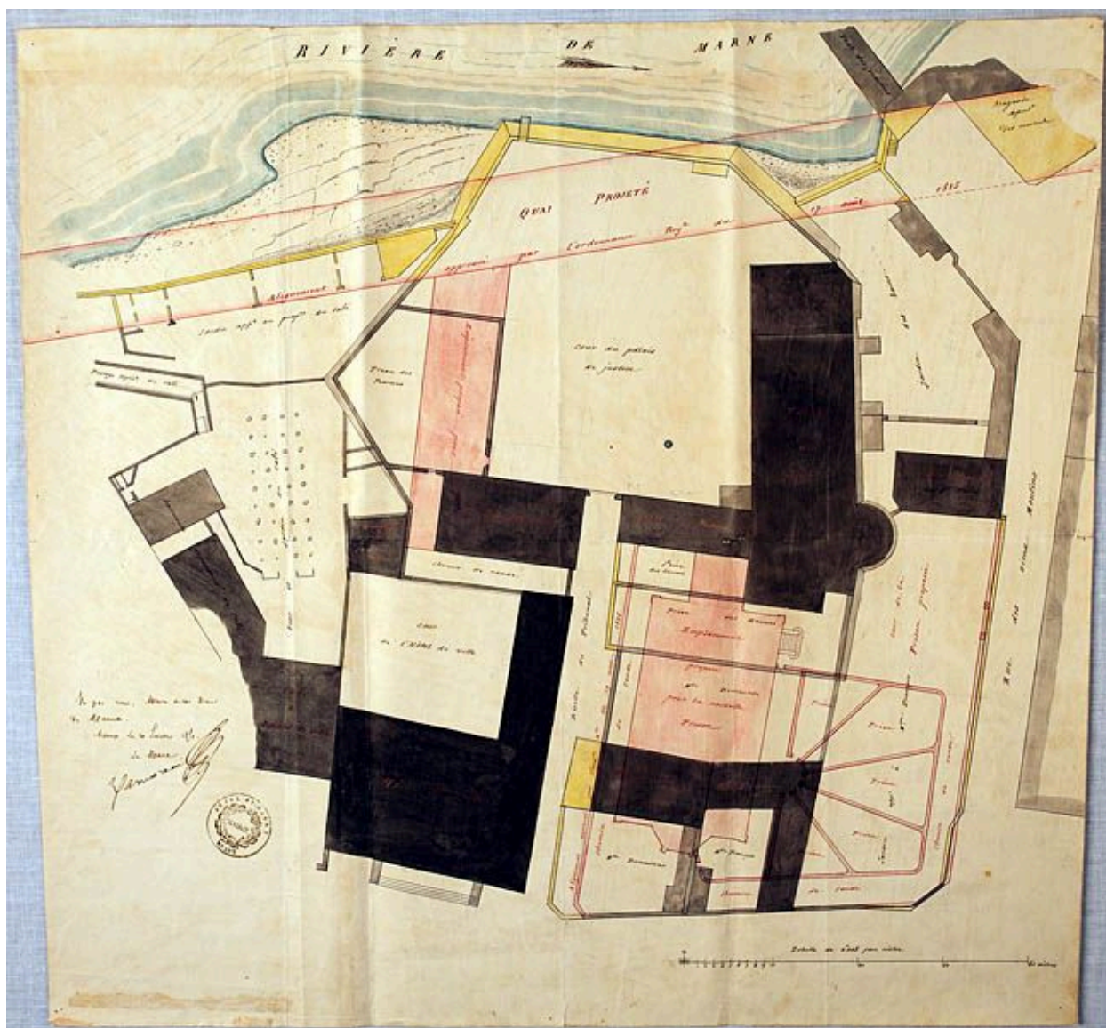
Plan de situation de l'ancien château des comtes de Champagne, avec le quai et la maison d'arrêt en projet en 1850. Papier aquarellé. (AD Seine-et-Marne. 4 N 110)
