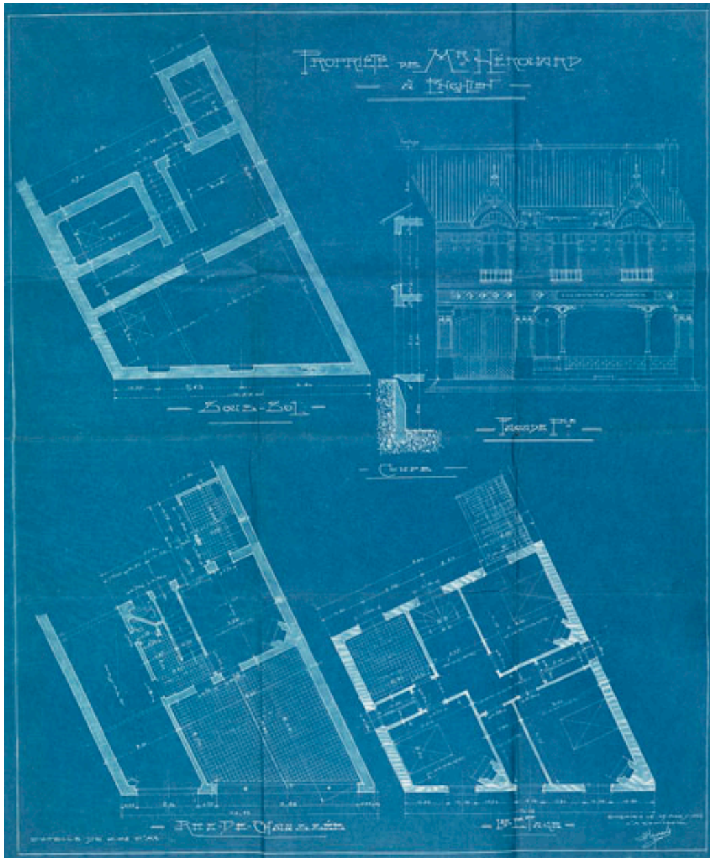
Elévation sur rue, plans des différents niveaux. (AM Enghien-les-Bains, Fonds des autorisations de permis de construire)
