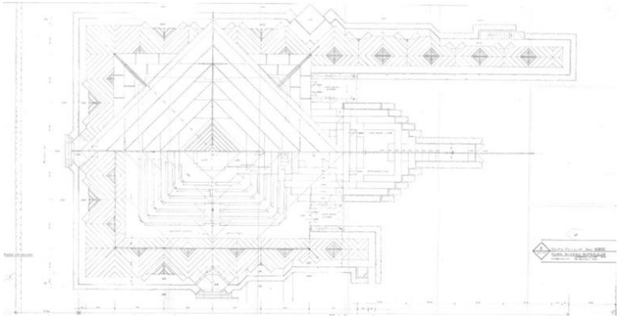
Plan niveau supérieur.
