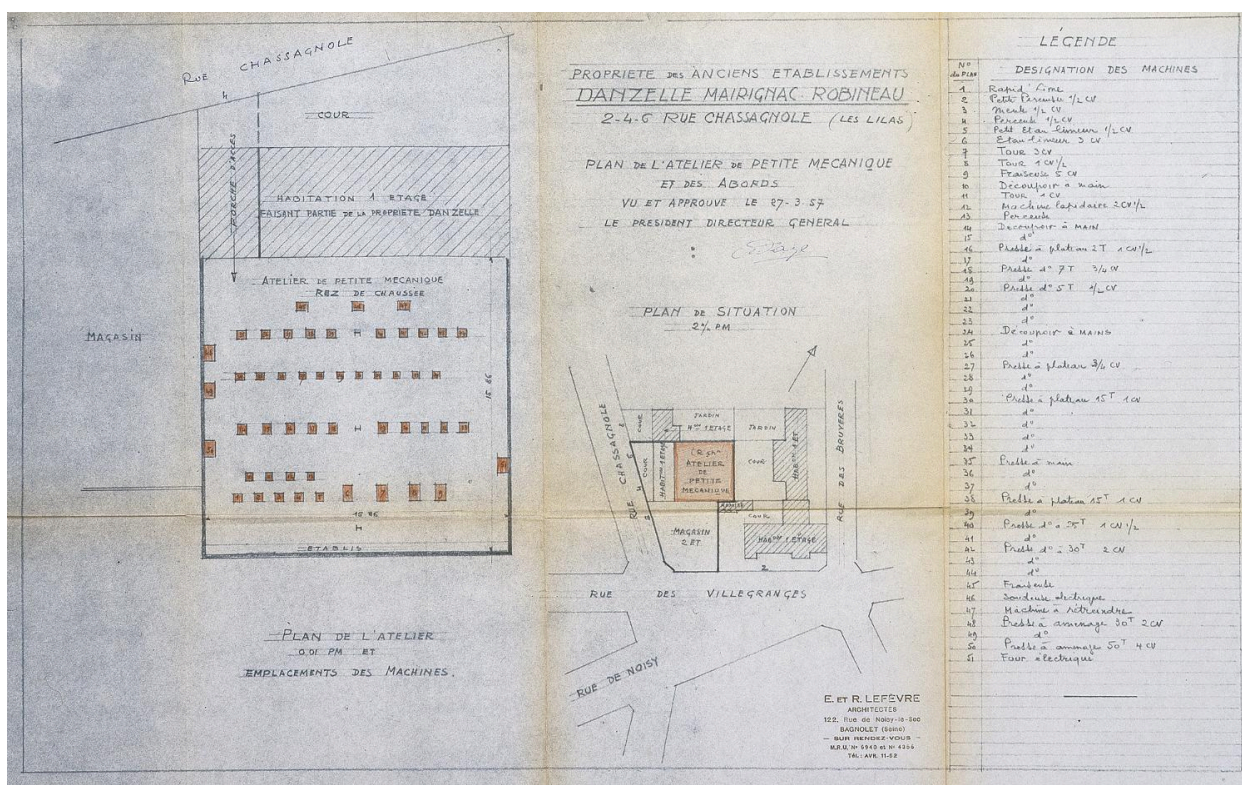
Plans de l'atelier de petite mécanique et de ses abords au 2-4-6 rue Chassagnolle, 1957 (AD93, 219 W 38).
