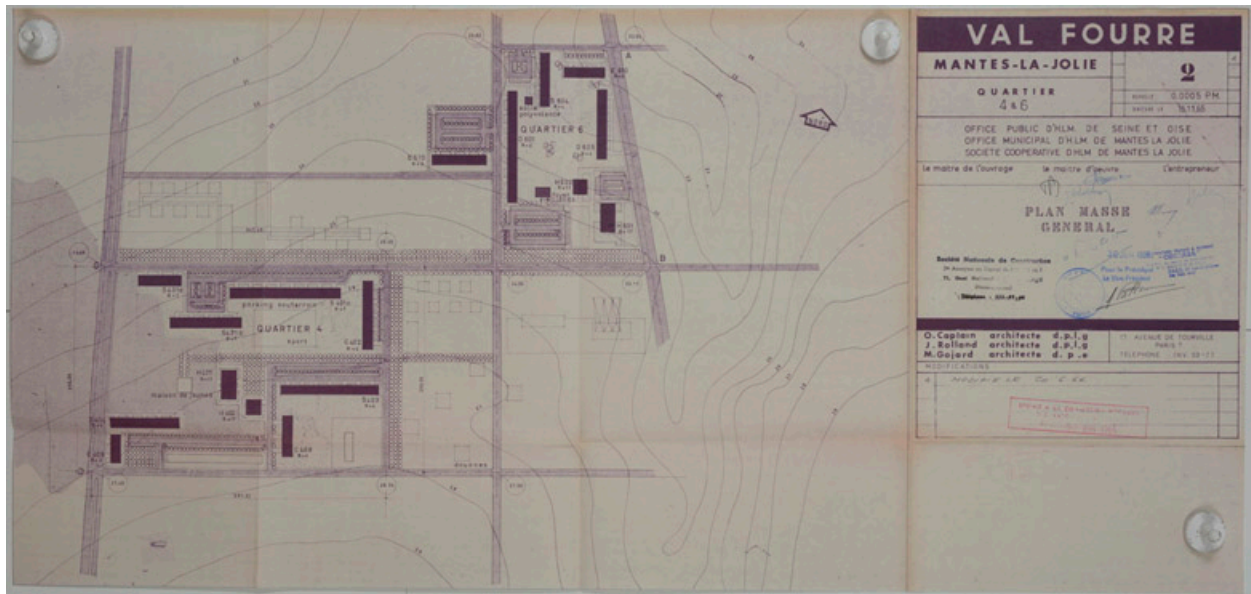
Quartiers 4 et 6 en 1965. Plan masse général. (Archives Nationales, Direction de l'Habitat et de la Construction, 19840091/130-132)
