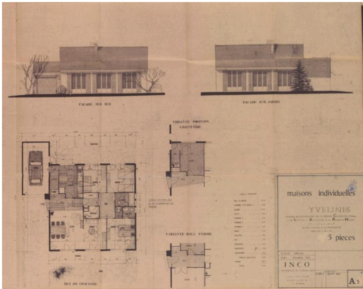
Quartier 7. Logements individuels et collectifs CLARM. Pavillon de 5 pièces. 1969. Mantes-la-Jolie, permis de construire 48/69.
